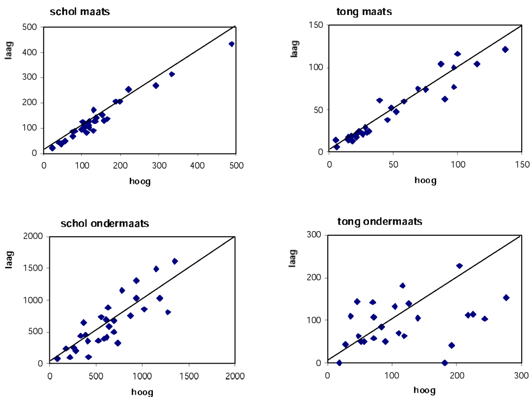
figuur 4. Vangst van maatse en ondermaatse tong en schol met de UK 153 als functie van de wekvelinstelling. Elk punt is 1 trek, waarbij met één tuig met een relatief sterk wekvel is gevisd. In geen van de gevallen is er een statistisch significant verschil in vangsten tussen beide instellingen (paired comparisons, Sokal & Rolpf, 1984), p < 0.05 .
