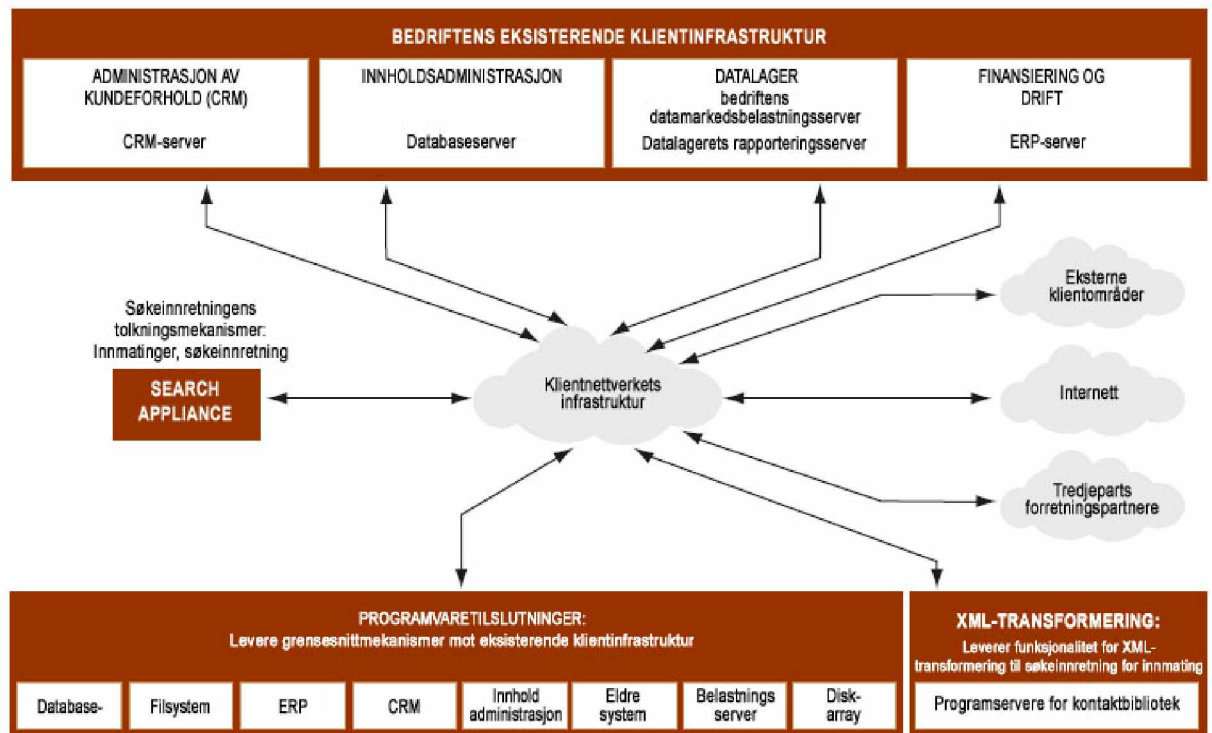
Figur 1. fysisk arkitektur på høyt nivå
