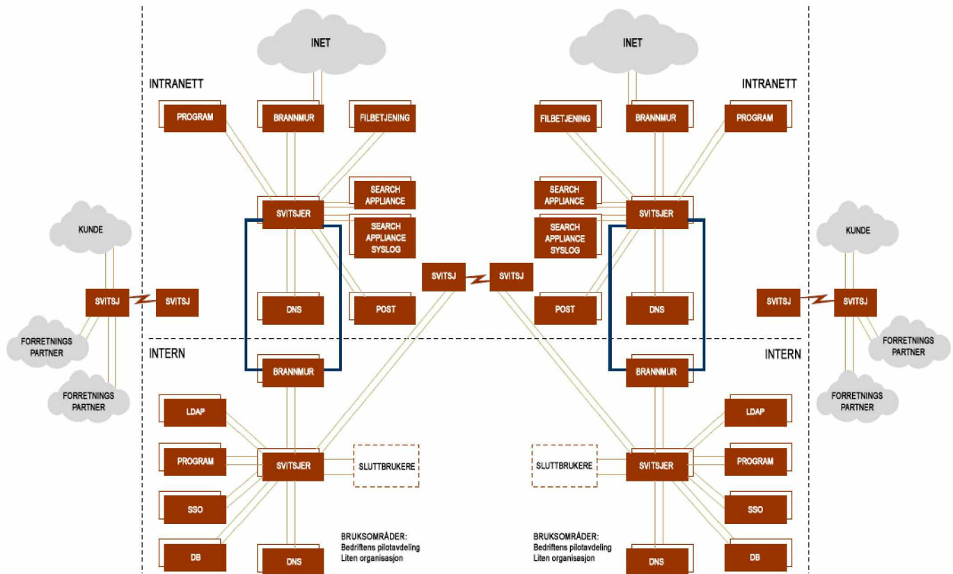
Figur 7. komplekst innføringsnettverk for en søkeløsning
